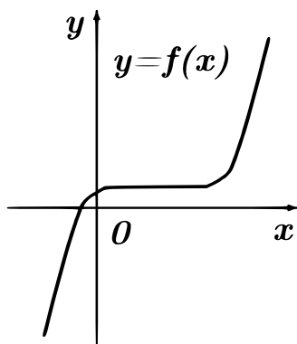
Рис. 5: Неубывающая функция
