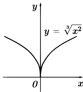
Рис. 8: f'(x_0) = \infty
