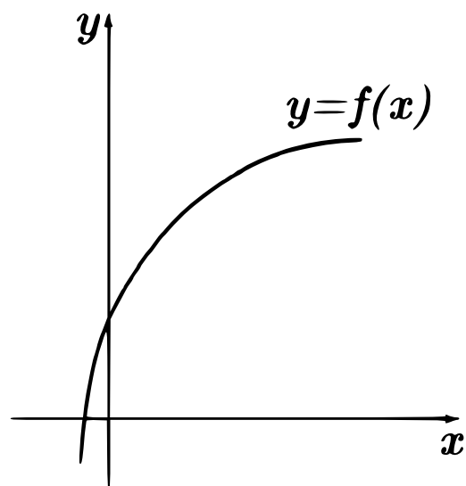
Рис. 13: Вогнутая функция
