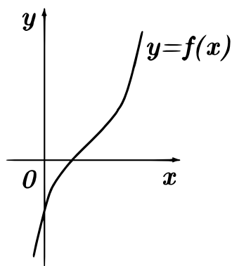
Рис. 5: Возрастающая функция
