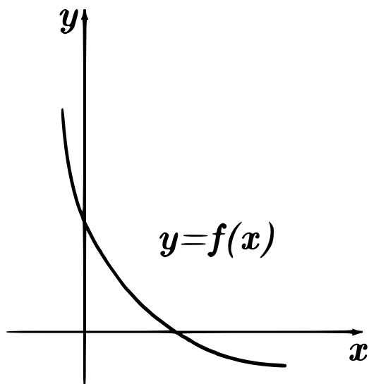
Рис. 12: Выпуклая функция
